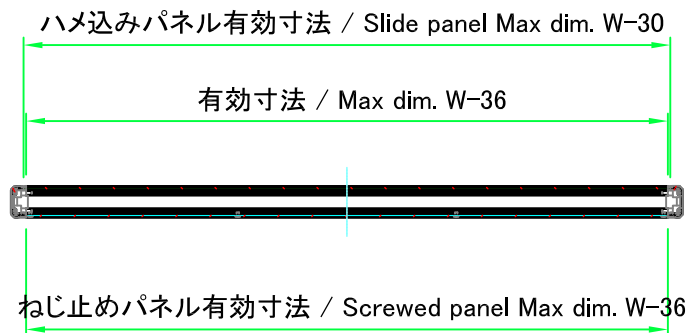
A-A (1:9)
